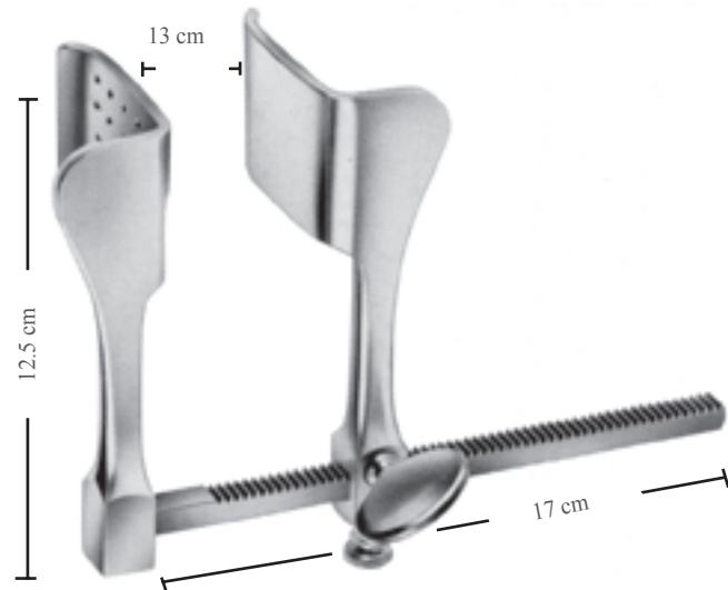
TUFFIER BM-7400 Göğüs ekartörü/Rib Retractor Bleydler/Blades 43 x 53 mm
