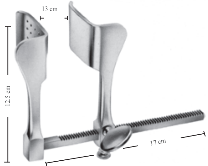
TUFFIER BM-7400 Göğüs ekartörü/Rib Retractor Bleydler/Blades 43 x 53 mm
