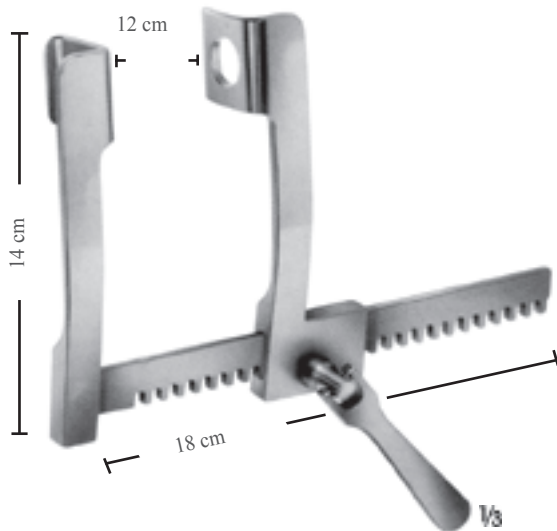
FINOCHIETTO BM-7700 Göğüs ekartörü/Rib retractor Bleydler/Blades 28 x 32 mm
