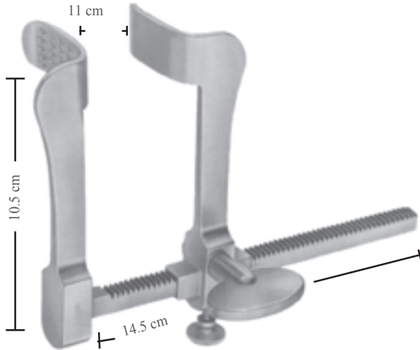
TUFFIER BM-7300 Bebekler için göğüs ekartörü Rib retractor for infants Bleydler/Blades 32 x 19 mm
