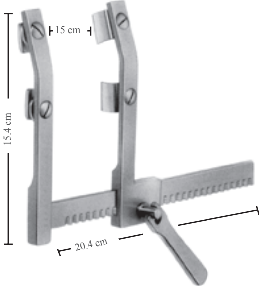
MORSE BM-8700 Sternum ayırıcı/Sternum spreaders Çocuklar için, hareket ettirilebilir çift bleydli For children with movable double blades Bleyd/Blade 12 x 20 mm
