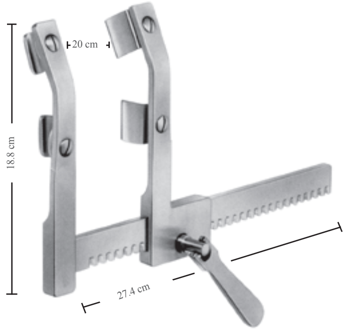
MORSE BM-8701 Sternum ayırıcı/Sternum spreaders Büyükler için, hareket ettirilebilir çift bleydler For adults with movable double blades Bleyd/Blade 19 x 29 mm
