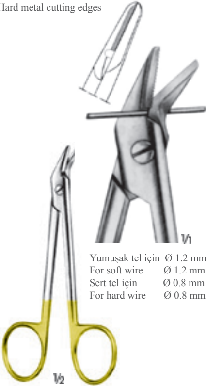
BC-7015 Tek ağız tırtıllı One jaw serrated 12 cm
