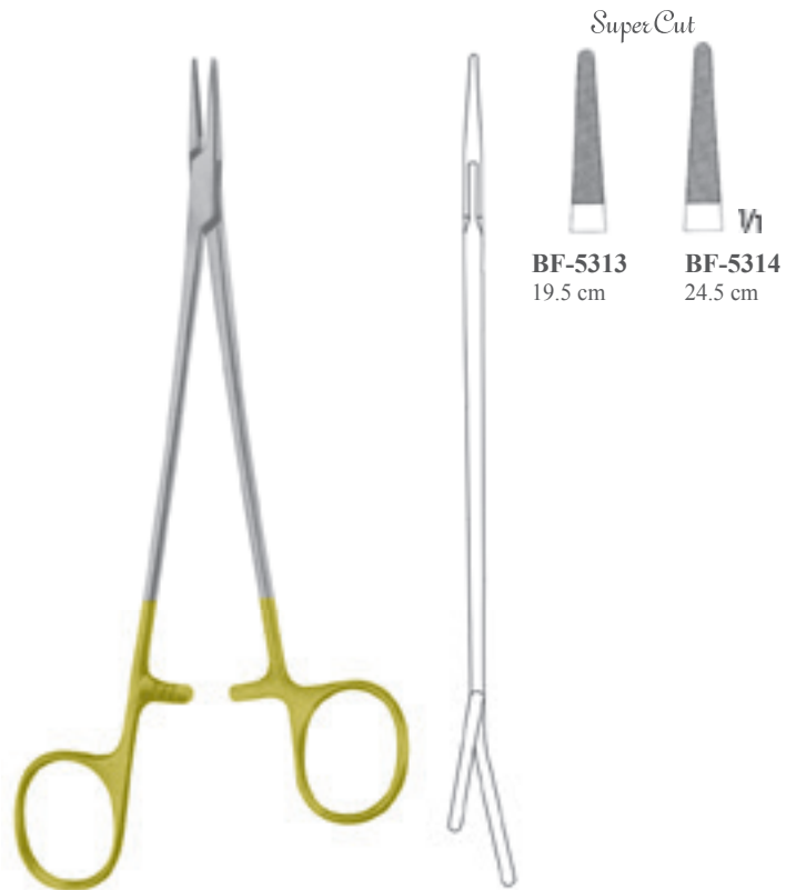
DE BAKEY BF-5313 - BF-5314 Uzatılmış bir sap ve kavisli yüzükler, optimum tutuş sağlar. One extended handle and curved rings ensure optimum grip
